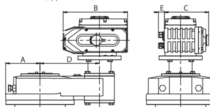
АМБ 160 (ЗДМ DN400)
