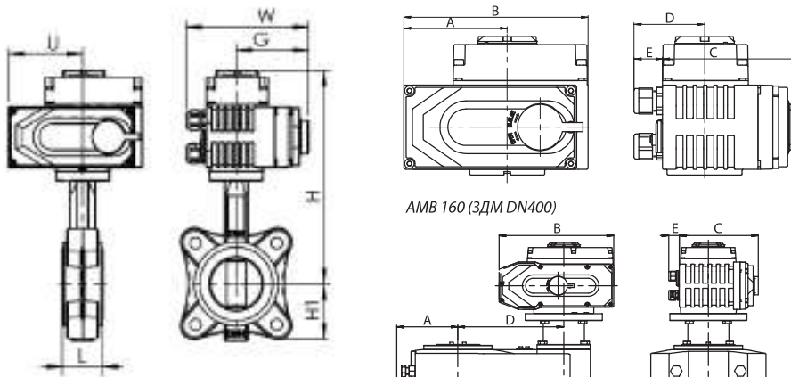
АМБ 003-100 (ЗДМ DN40–350)
